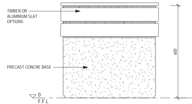
4 END ELEVATION 1: 10 @ A3
