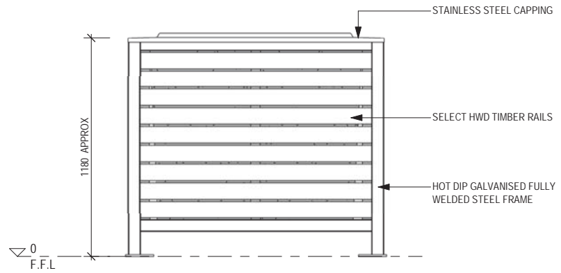
2 END ELEVATION 1:20 @ A3
