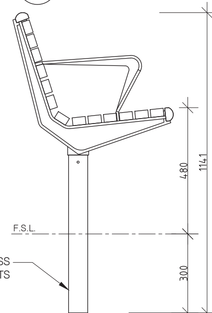
2 END ELEVATION 1:10 @ A3
