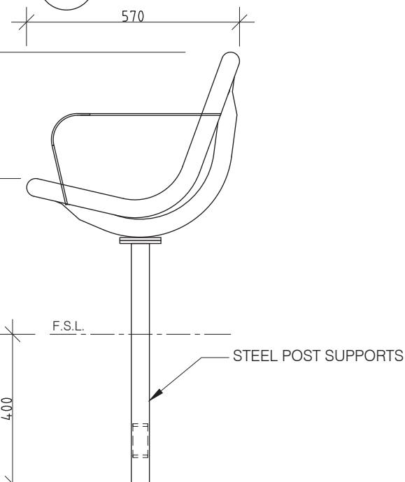
3 END ELEVATION 1:10 @ A3
