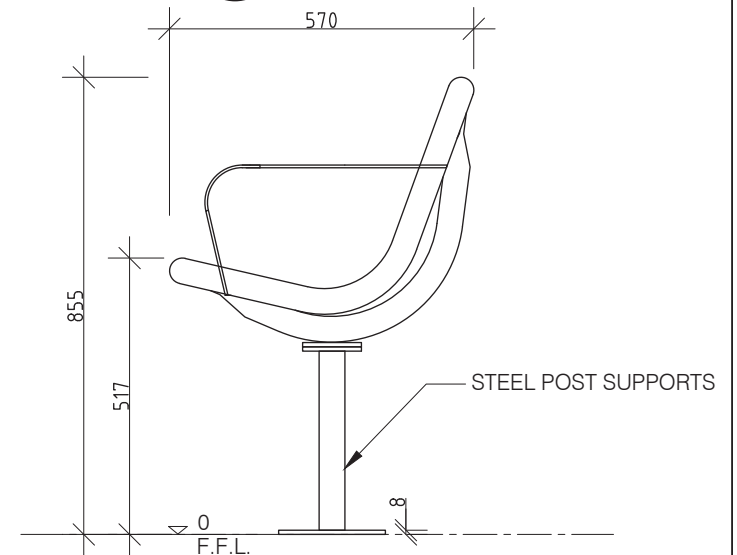
3 END ELEVATION 1:10 @ A3
