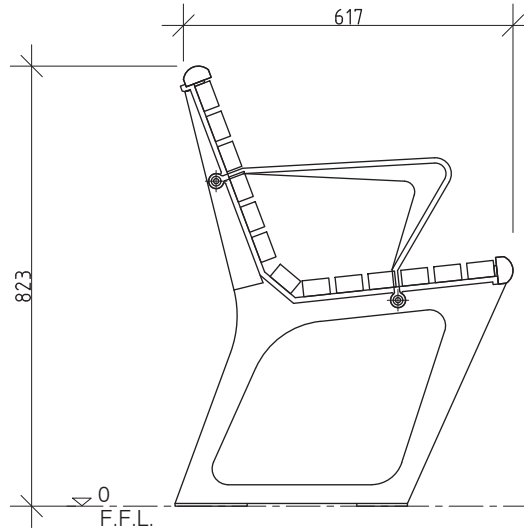
2 END ELEVATION 1:10 @ A3
