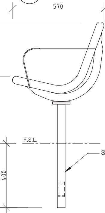
3 END ELEVATION 1:10 @ A3
