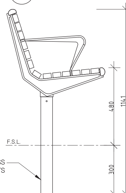
2 END ELEVATION 1:10 @ A3
