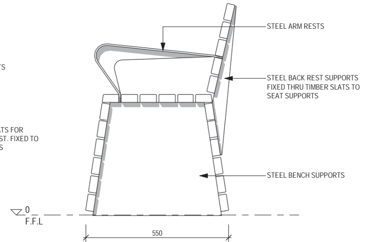
2 END ELEVATION 1:10 @ A3
