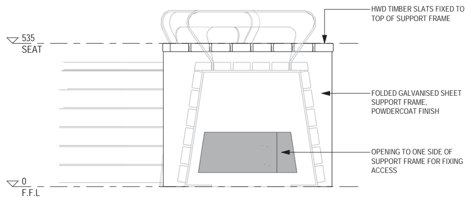
2 END ELEVATION 1 : 10 @ A3
