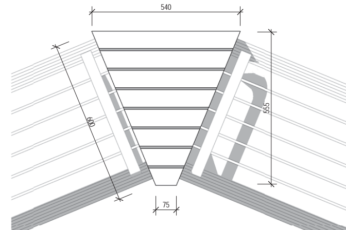
5 PLAN 001 1 : 10 @ A3
