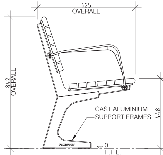
2 END ELEVATION 1:10 @ A3
