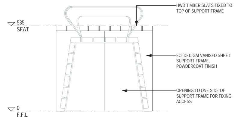
2 END ELEVATION 1:10 @ A3
