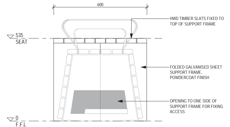
2 END ELEVATION 1:10 @ A3
