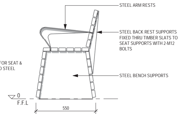
2 END ELEVATION 1:15 @ A3
