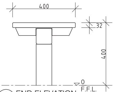
3 END ELEVATION 1:10 @ A3
