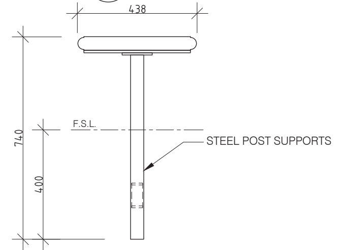
3 END ELEVATION 1:10 @ A3
