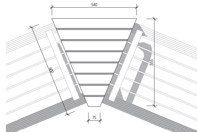
5 PLAN 001 1 : 10 @ A3
