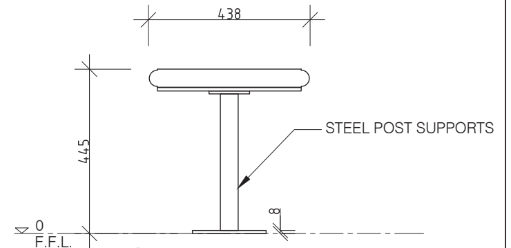
3 END ELEVATION 1:10 @ A3
