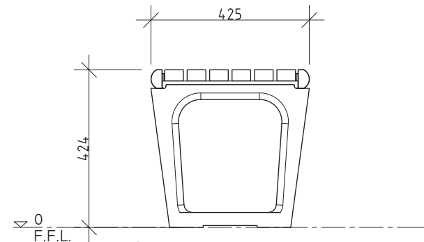
3 END ELEVATION 1:10 @ A3
