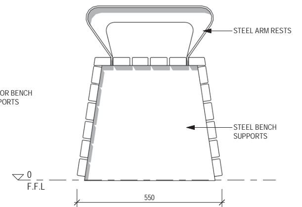
2 END ELEVATION
