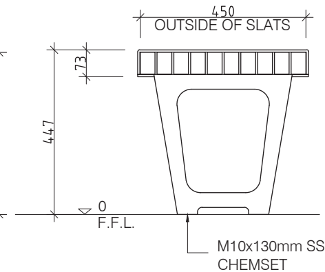
3 END ELEVATION 1:10 @ A3
