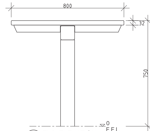
3 END ELEVATION 1:10 @ A3
