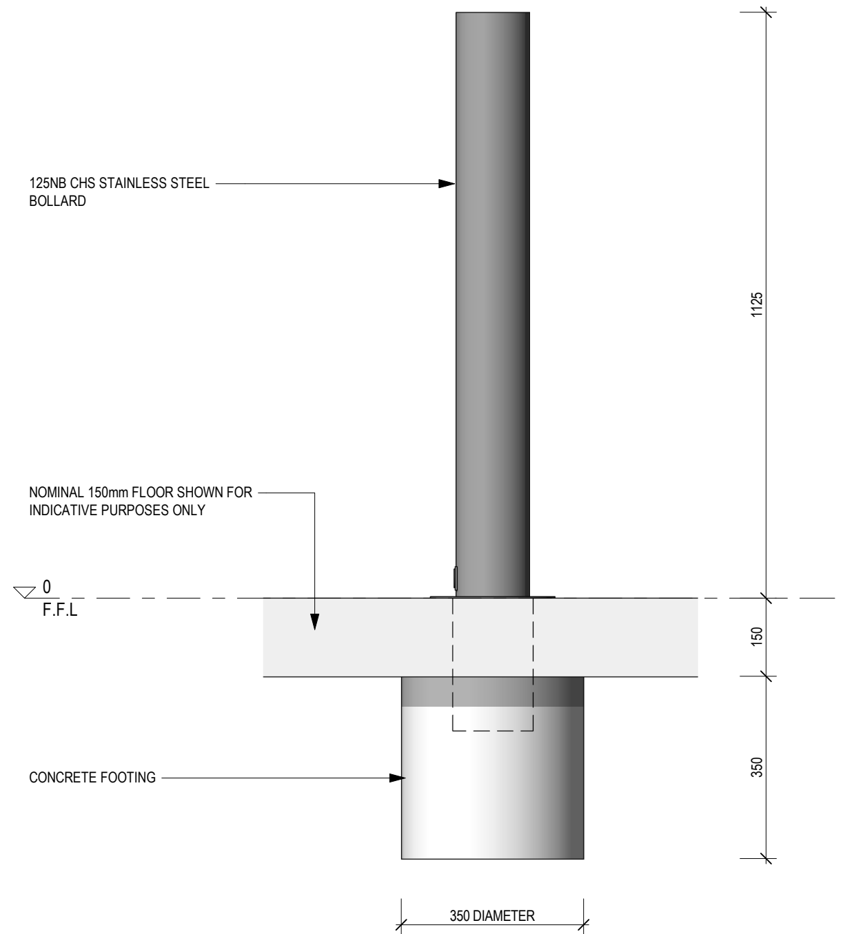
1 BOLLARD ELEVATION 1:10 @ A3
